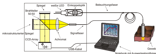
Abb. 2 Messaufbau des Fourierspektrometers am Beispiel eines Blutanalysestystems
