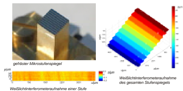
Abb. 5 mikrostrukturierter Stufenspiegel
