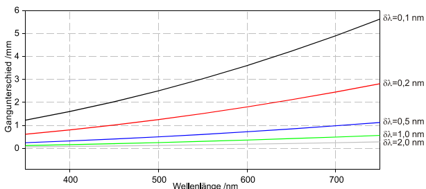
Abb. 3 erforderlicher Gangunterschied
