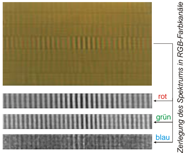
Abb. 4 Fourierspektrum einer Gasentladungslampe
