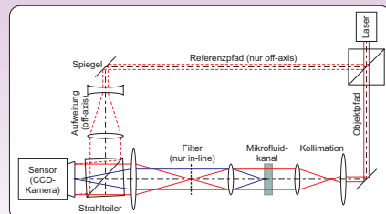
Bild 2: Holografische Versuchsanordnung
